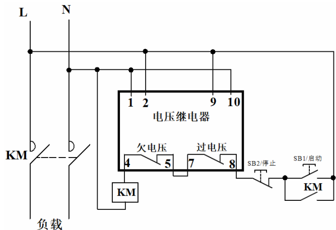
过、欠电压保护应用案例
