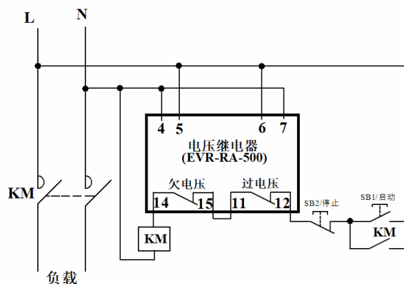
单相过、欠电压保护应用实例（工作方式 1）
