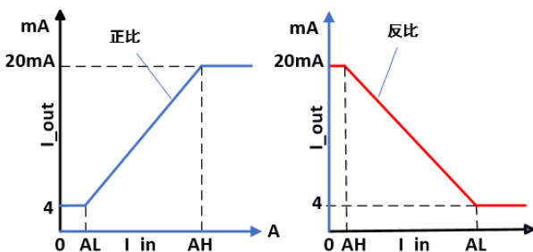
输入电流和输出电流关系：
