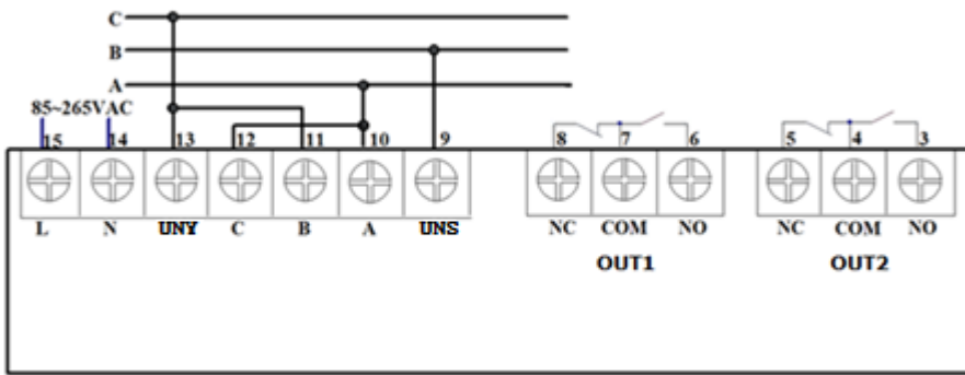
三相三线制接线
