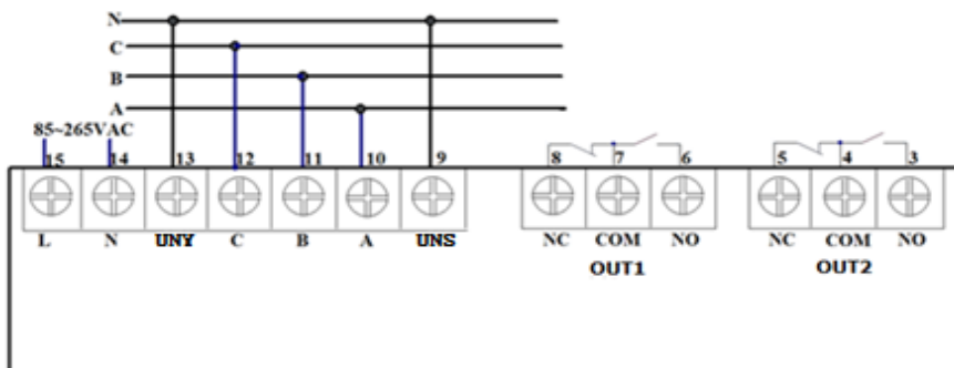
三相四线制接线
